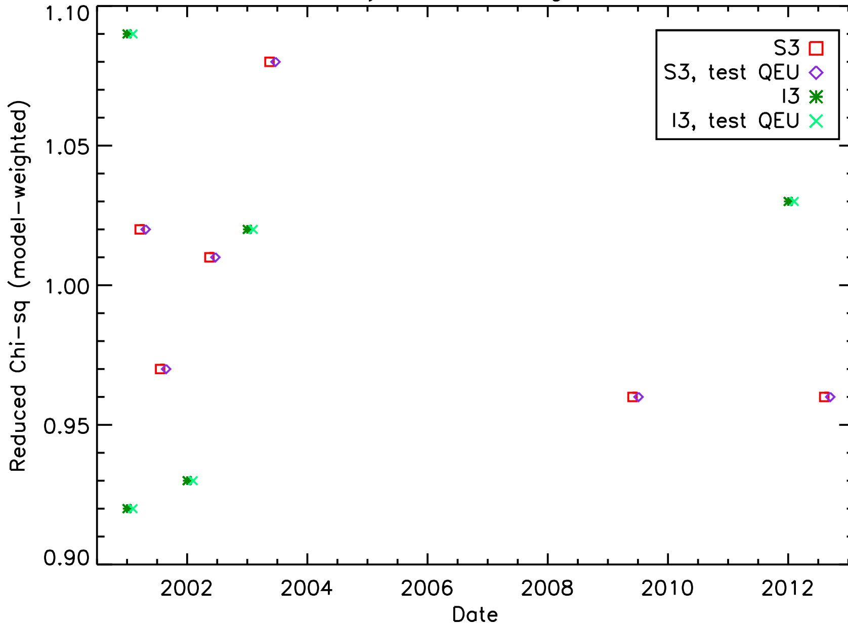
ACIS subarray G21.5-0.9 goodness of fit
